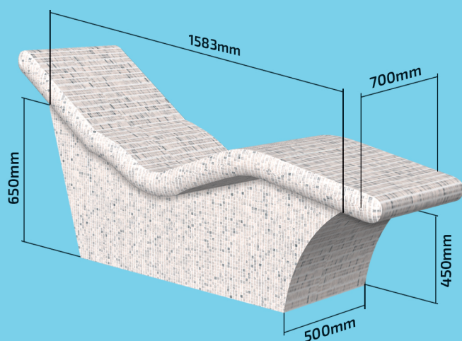
MEGA TEPIDARIJUM - TOPLA LEŽALJKA "A"
