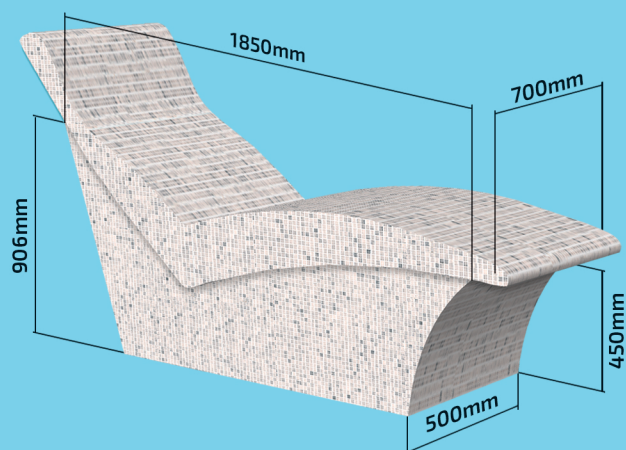
MEGA TEPIDARIJUM - TOPLA LEŽALJKA "B"
