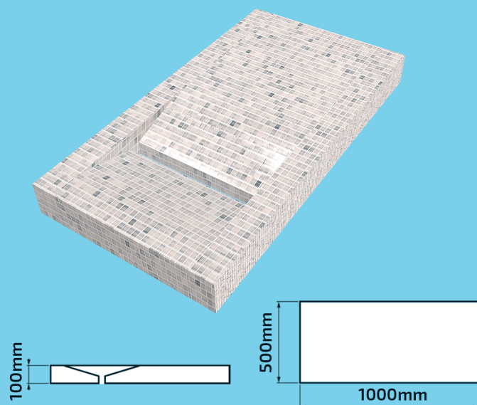
MEGA UMIVAONIK B
